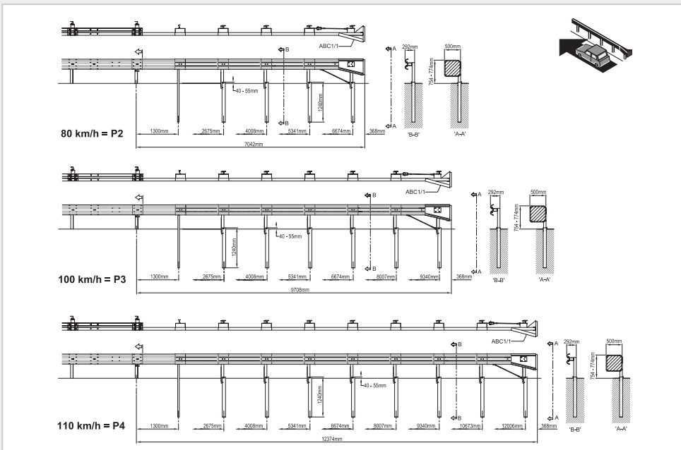
Schemat 3. Sposób montażu Terminalu ABC wówczas, gdy odcinek końcowy znajduje się po prawej stronie ruchu drogowego
