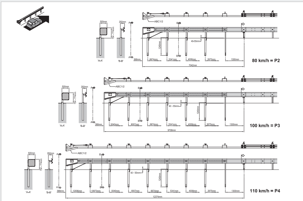
Schemat 2. Sposób montażu Terminalu ABC wówczas, gdy odcinek końcowy znajduje się po lewej stronie ruchu drogowego
